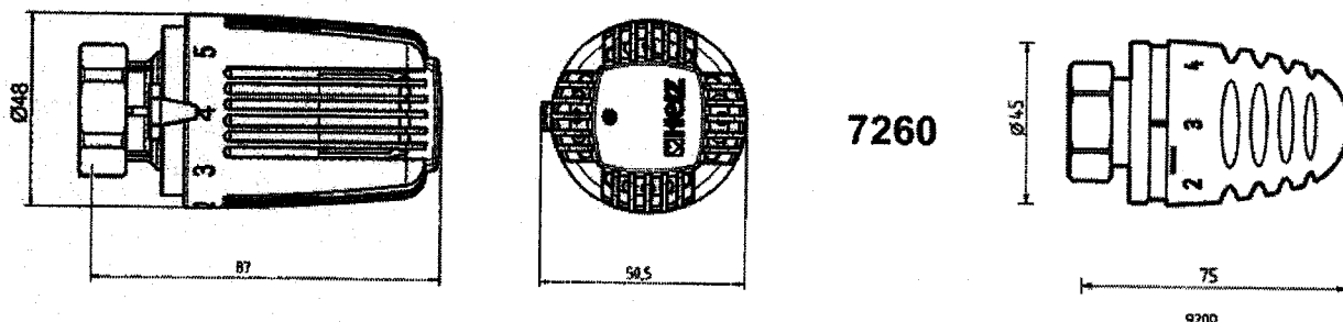
Slika 1. Izgled i dimenzije termostatskih glava STANDARD i MINI artikl br.7260 i 9200
