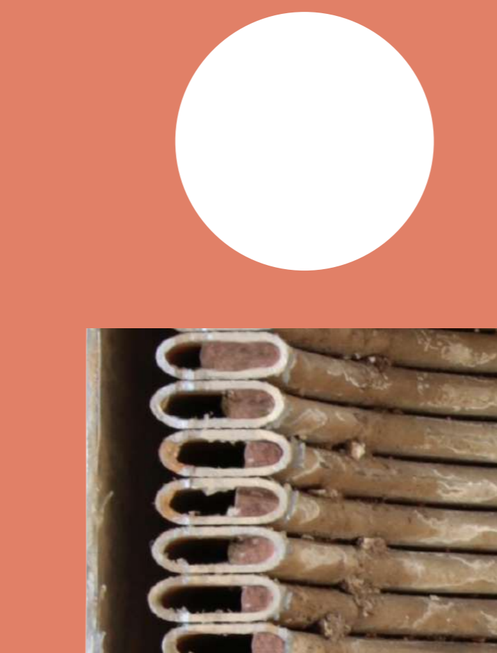
IZMENJIVAČ TOPLOTE KONDENZACIONOG KOTLA - PRESEK KALEMA
