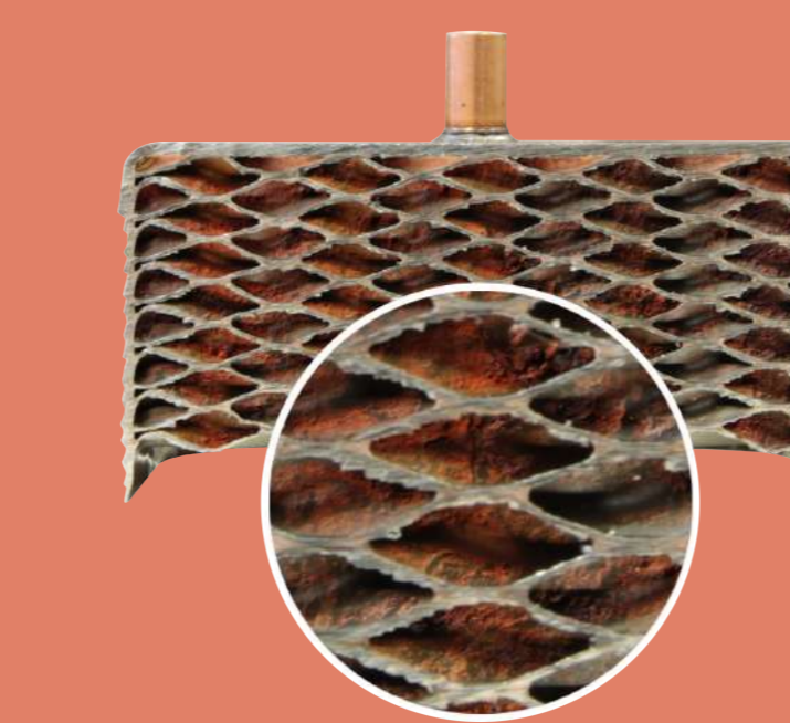
IZMENJIVAČ TOPLOTE KONDENZACIONOG KOTLA - PRESEK KALEMA
