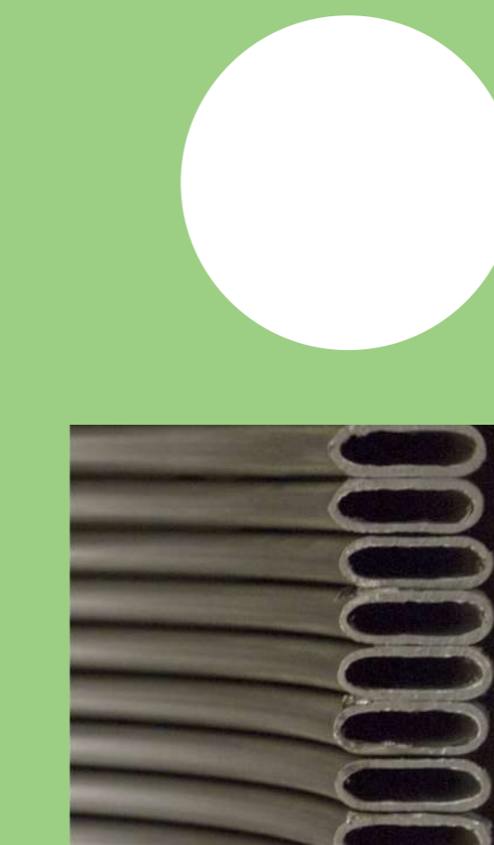
IZMENJIVAČ TOPLOTE KONDENZACIONOG KOTLA - PRESEK KALEMA
